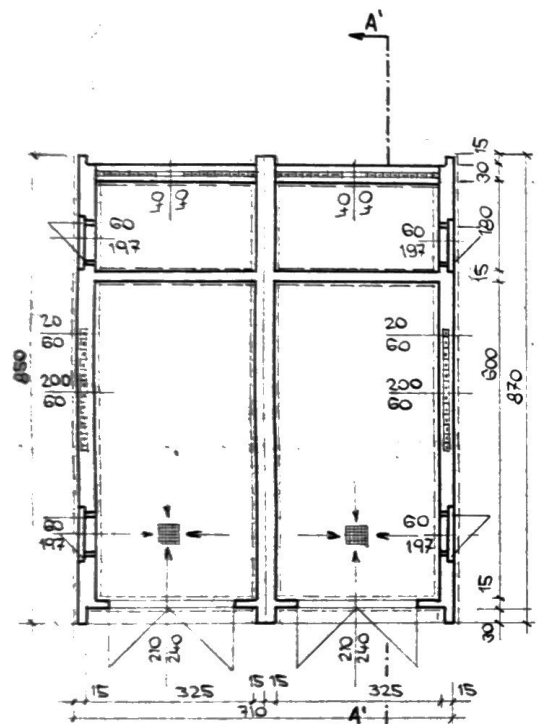
PŮDORYS 1:100
